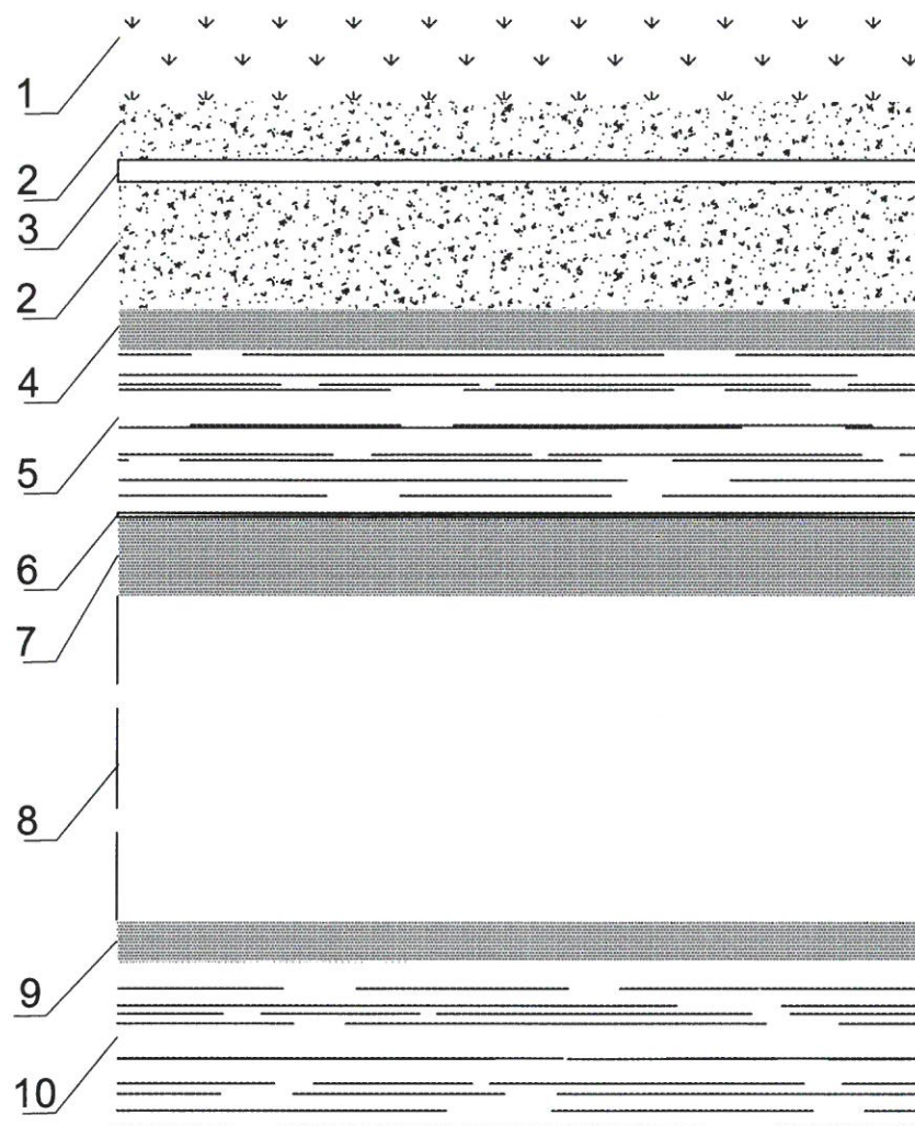
PRZEKRÓJ PODŁUŻNY
